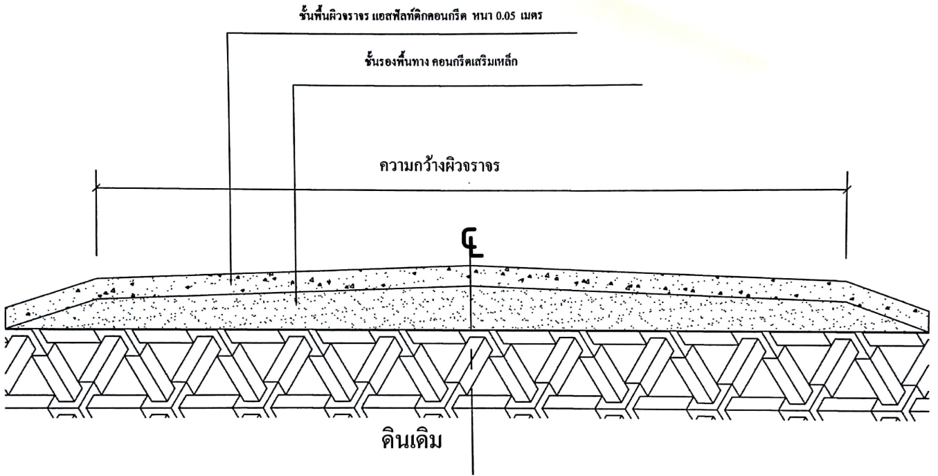
แสดงแบบรูปตัดถนน เสริมผิวจราจรแอสฟัลต์ติกคอนกรีต
