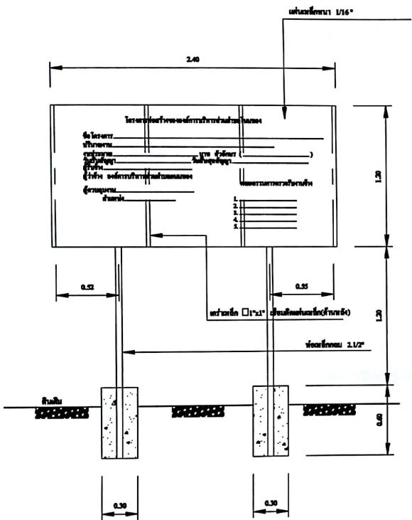
แบบเขียนประกอบขึ้นโครงตามรูปที่ ๑ มาตราส่วน 1 : 30
