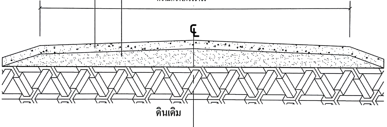
แสดงแบบรูปตัดถนน เวิรมิผิวจราจรแอสฟัลต์ติกคอนกรีต
